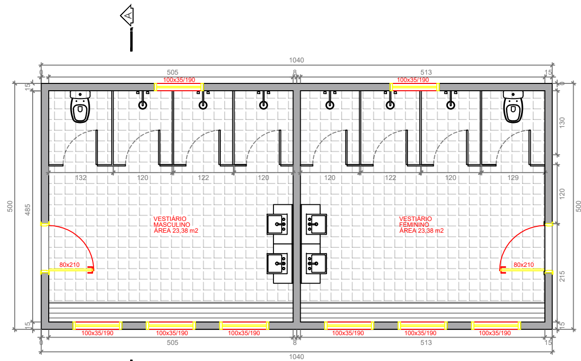
PLANTA BAIXA VESTIÁRIOS
